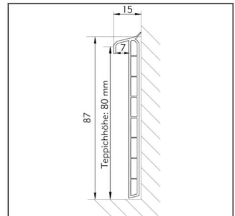
Abb. 2: Maßzeichnung HZ-Teppich-Blindleiste BLT
