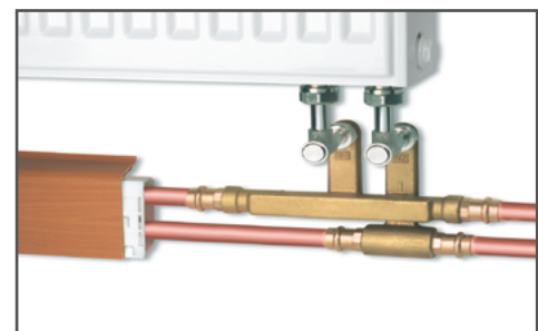
Abb. 5: HZ-Heizkörperanschluss
