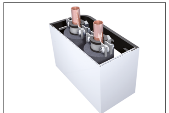
Abb. 9: HZ-Steigstrangprofil
